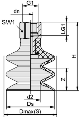
Tasarım verileri FSG 14 NBR-55 G1/8-IG
