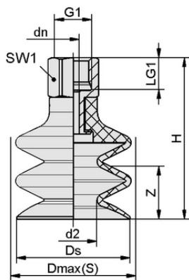
Datos de diseño FSG 14 NBR-55 G1/8-IG
