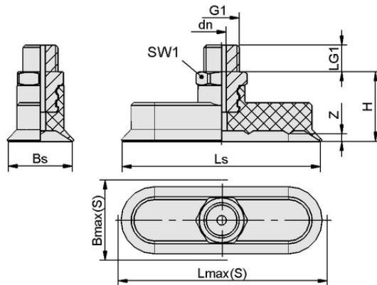
デザインデータ SGON 30x10 SI-HD-65 G1/8-AG
