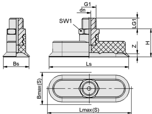
デザインデータ SGON 4x2 NBR-ESD-55 M3-AG
