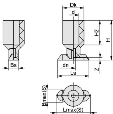
Données de construction SGO 12x4 NBR-ESD-55 N020
