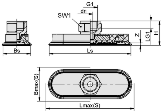
Datos de diseño SAOF 80x40 NBR-45 NPT3/8-IG
