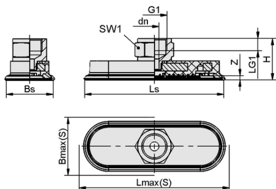
デザインデータ SAOF 80x40 HT2-65 G1/4-IG
