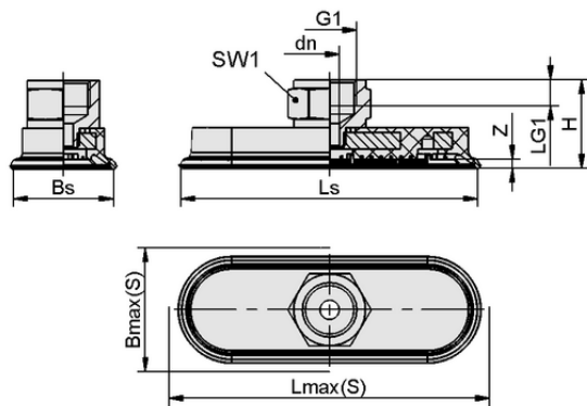
Datos de diseño SAOF 80x40 HT2-65 G1/4-IG
