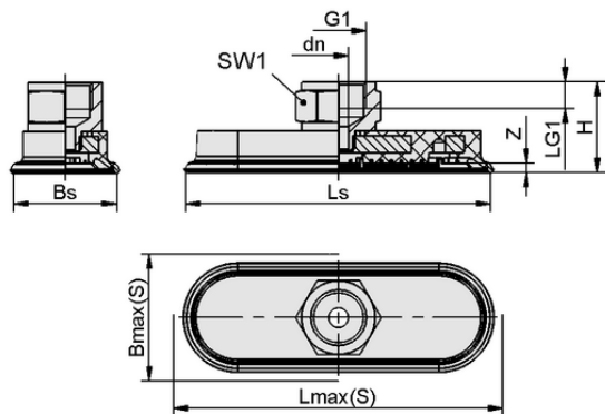
Datos de diseño SAOF 90x30 HT2-65 G3/8-IG
