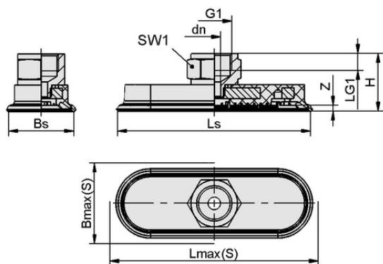
Конструктивные данные SAOF 140x70 NBR-45 G3/8-IG
