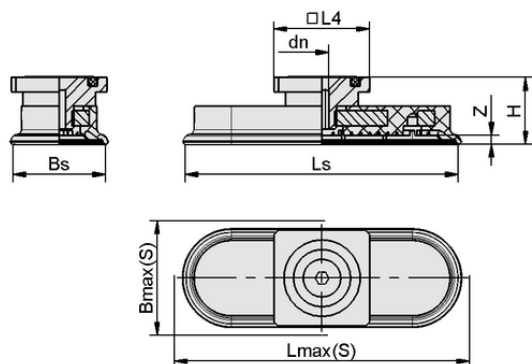
デザインデータ SAOF 120x60 NBR-45 RA
