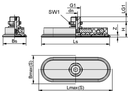
Données de construction SAOF 120x60 NBR-45 G1/4-AG
