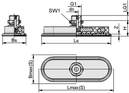
Tasarım verileri SAOF 80x40 NBR-45 M10-AG
