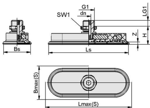
デザインデータ SAOF 80x40 NBR-45 M10-AG
