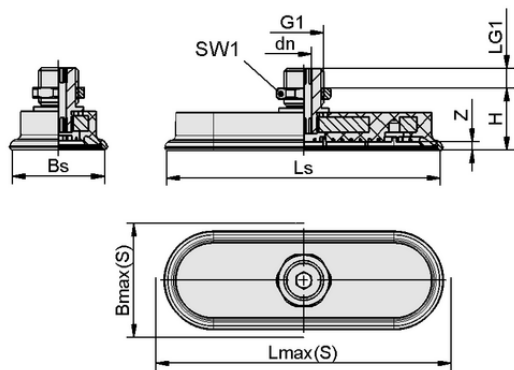
Design data SAOF 80x40 NBR-45 M10-AG
