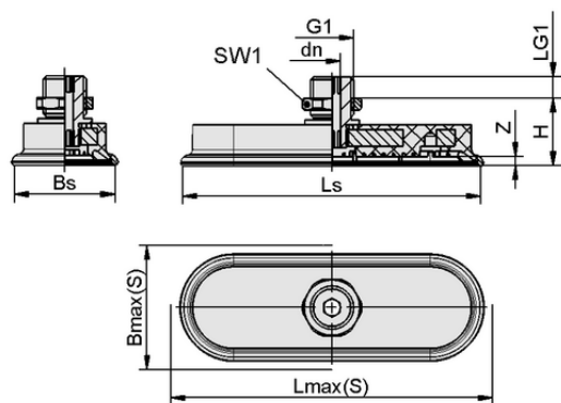
Datos de diseño SAOF 80x40 NBR-45 M10-AG
