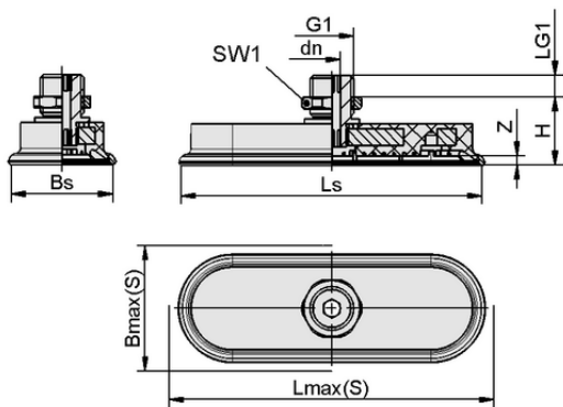
Données de construction SAOF 80x40 NBR-45 M10-AG
