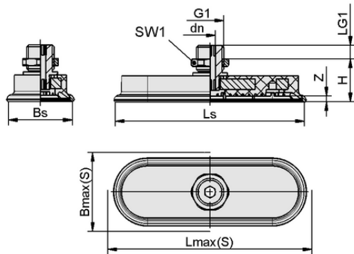
Datos de diseño SAOF 80x40 NBR-45 G1/4-AG
