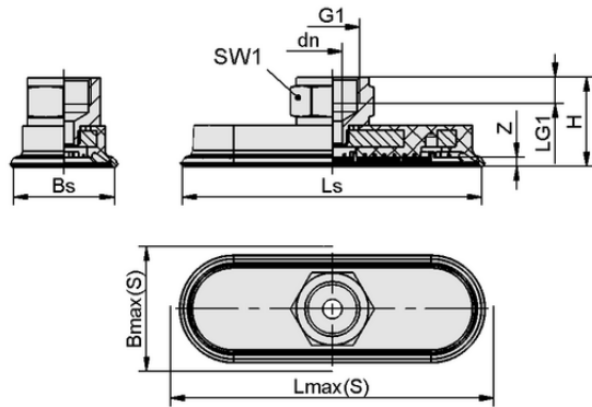
Datos de diseño SAOF 90x30 NBR-45 G3/8-IG
