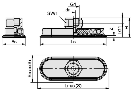
Données de construction SAOF 90x30 NBR-45 G1/4-IG
