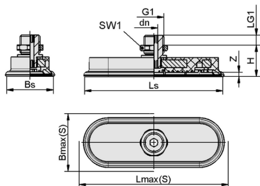
デザインデータ SAOF 50x16 NBR-45 M10-AG
