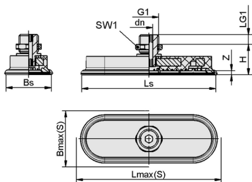
Конструктивные данные SAOF 50x16 NBR-60 M14x1.5-AG
