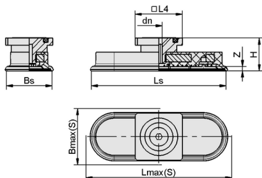
デザインデータ SAOF 50x16 NBR-60 RA
