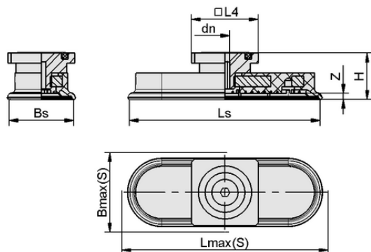
Конструктивные данные SAOF 50x16 NBR-60 RA
