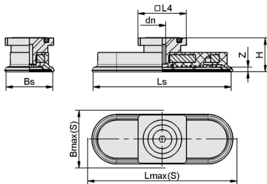
Datos de diseño SAOF 50x16 NBR-60 RA
