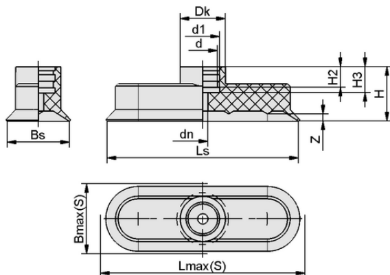
Datos de diseño SGO 30x10 HT1-60 N022
