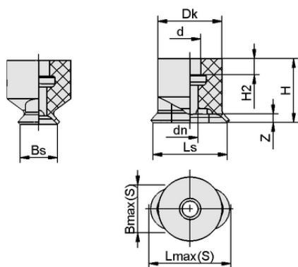
Конструктивные данные SGO 7x3.5 HT1-60 N003
