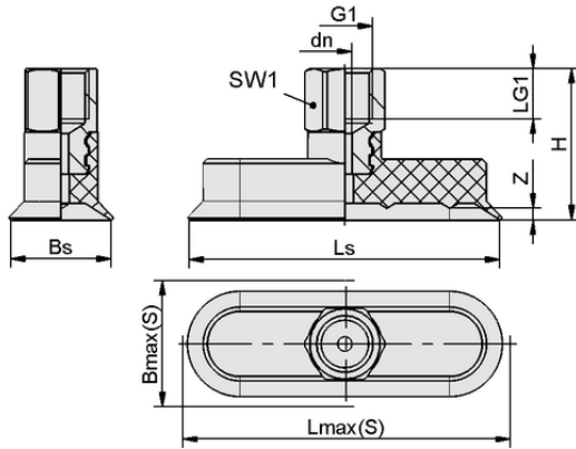
Tasarım verileri SGON 24x8 HT1-60 G1/8-IG
