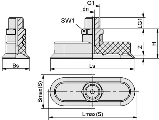
Tasarım verileri SGON 24x8 HT1-60 G1/8-AG
