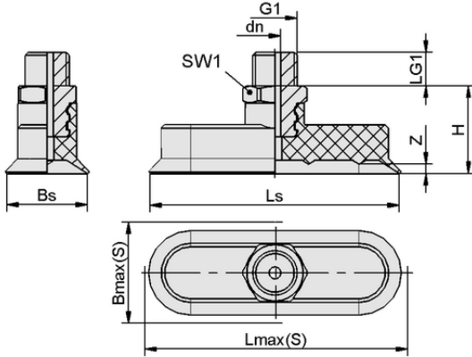
Tasarım verileri SGON 15x5 HT1-60 M5-AG
