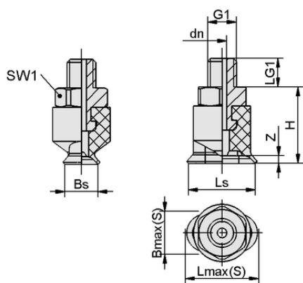
Конструктивные данные SGON 4x2 HT1-60 M3-AG
