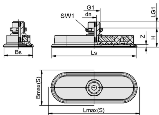
Конструктивные данные SAOF 60x23 NBR-60 M10-AG
