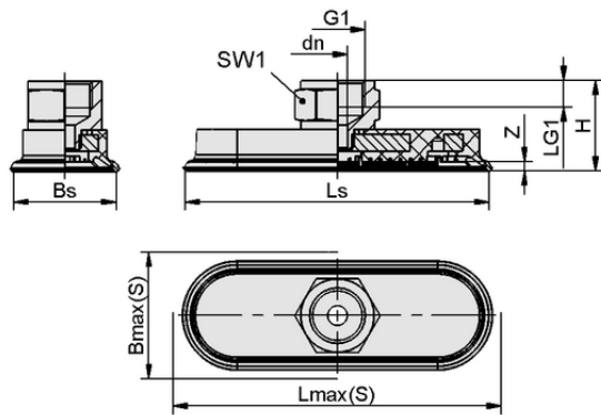
Datos de diseño SAOF 60x23 NBR-60 G3/8-IG
