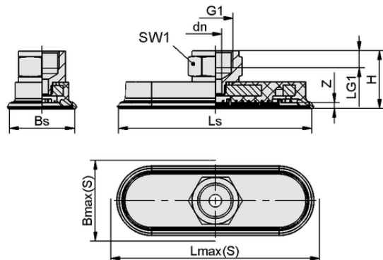
デザインデータ SAOF 60x23 NBR-60 G3/8-IG
