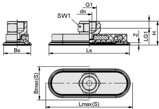
Datos de diseño SAOF 60x23 NBR-60 G1/4-IG
