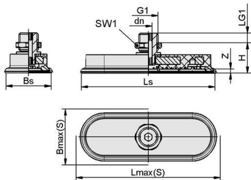
Datos de diseño SAOF 140x70 NBR-60 M14x1.5-AG
