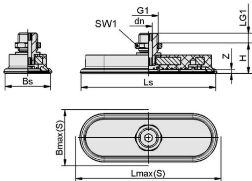
Données de construction SAOF 100x50 NBR-60 G1/4-AG
