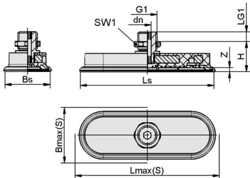
Datos de diseño SAOF 100x50 NBR-60 G1/4-AG
