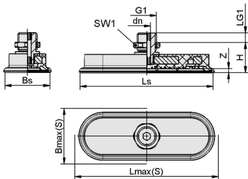
デザインデータ SAOF 80x40 NBR-60 G1/4-AG
