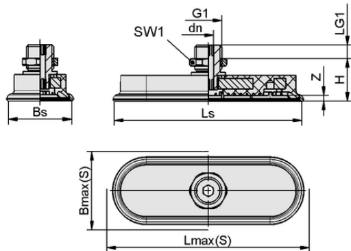
Datos de diseño SAOF 90x30 NBR-60 G1/4-AG
