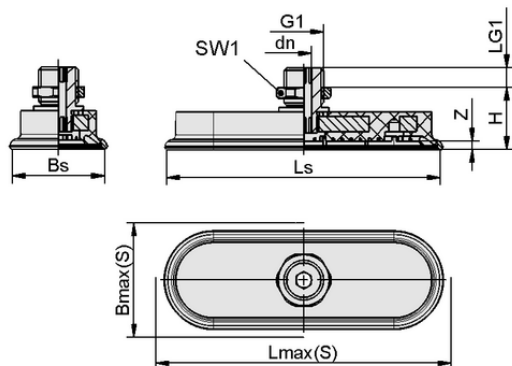
Données de construction SAOF 90x30 NBR-60 G1/4-AG
