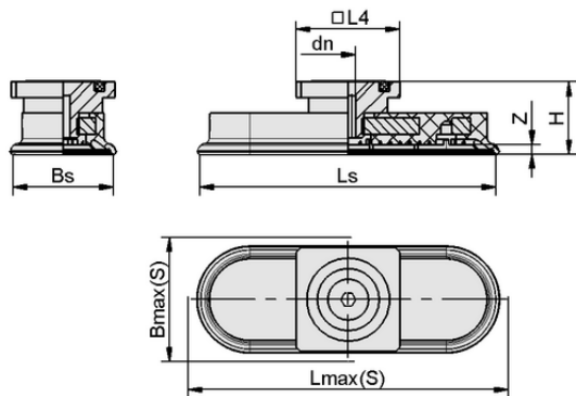
Données de construction SAOF 80x40 NBR-60 RA
