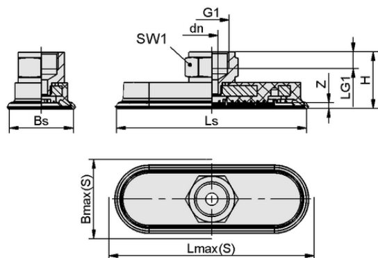
Datos de diseño SAOF 80x40 NBR-60 G3/8-IG
