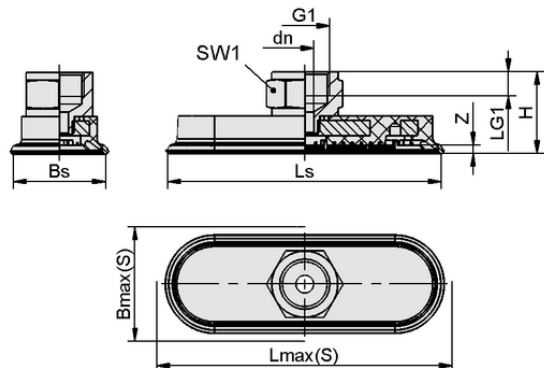
デザインデータ SAOF 80x40 NBR-60 G3/8-IG
