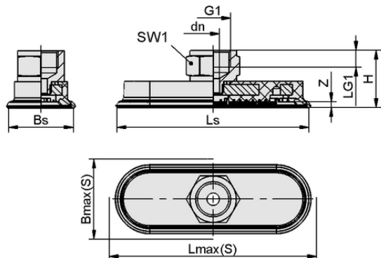
Données de construction SAOF 90x30 NBR-60 G3/8-IG
