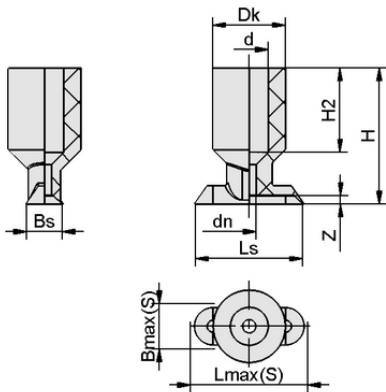
Datos de diseño SGO 12x4 NBR-CO-55 N020
