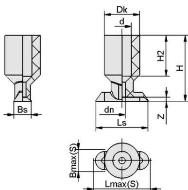
Dati di costruzione SGO 15x5 NBR-CO-55 N021
