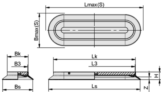
Datos de diseño SPLO 300x55 NBR-55
