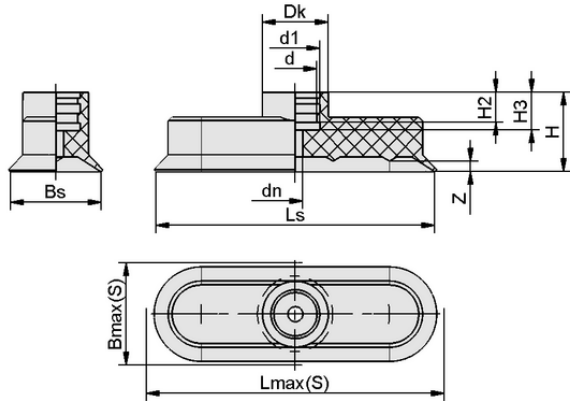
Tasarım verileri SGO 30x10 NBR-55 N022
