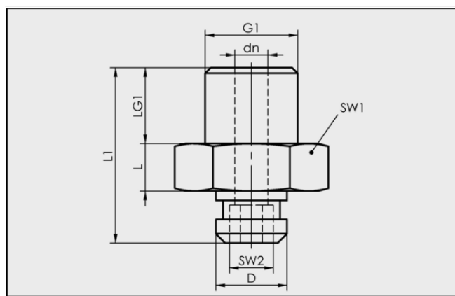
Datos de diseño SA-NIP N021 M5-AG DN200
